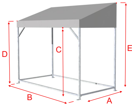
SECTIONS DE LA STRUCTURE Tube carré acier électrozingué 40x40x2
